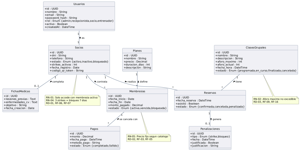
Figura 2.4: Diagrama de Clases del Dominio — Modelo de Datos OLYMPUS CORE (MVP1)
