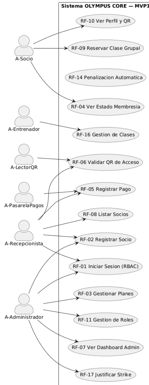
Diagrama de Casos de Uso — Nivel de Sistema (Funcionalidades que el sistema OLYMPUS CORE automatizara)
