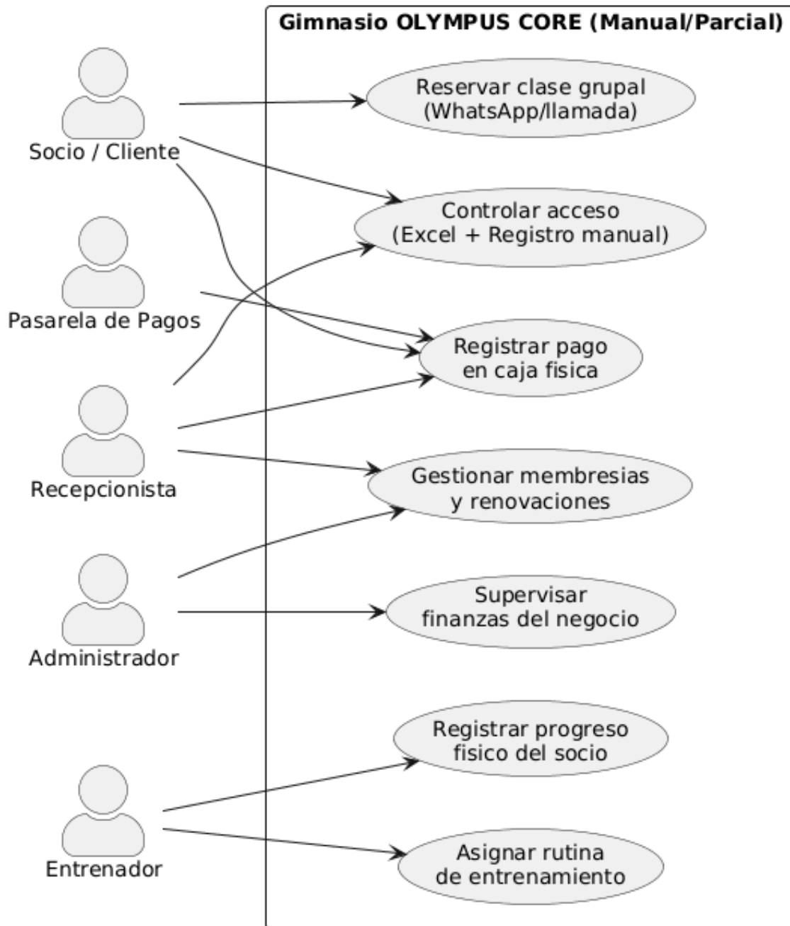
Figura 1.7: DCU Nivel de Negocio — Procesos del dominio OLYMPUS CORE
